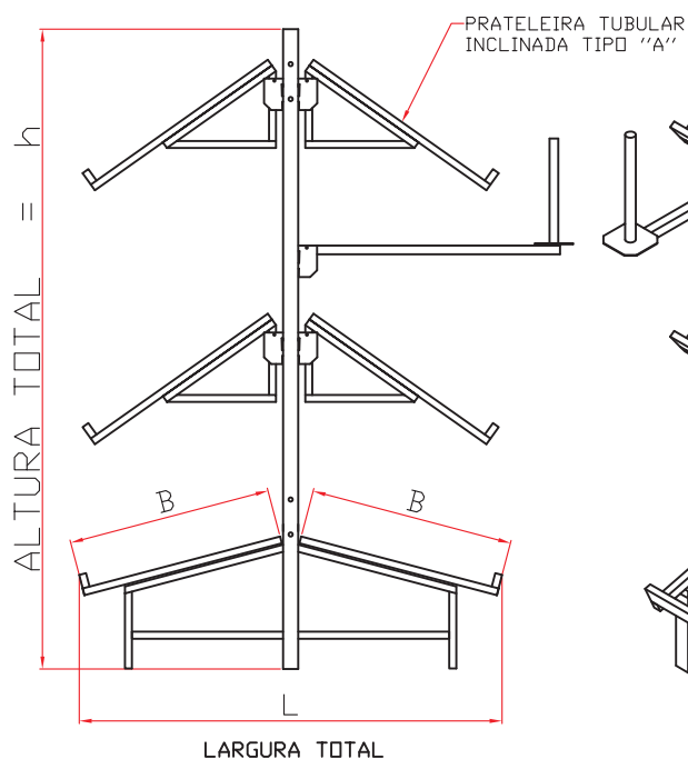
CORTE
